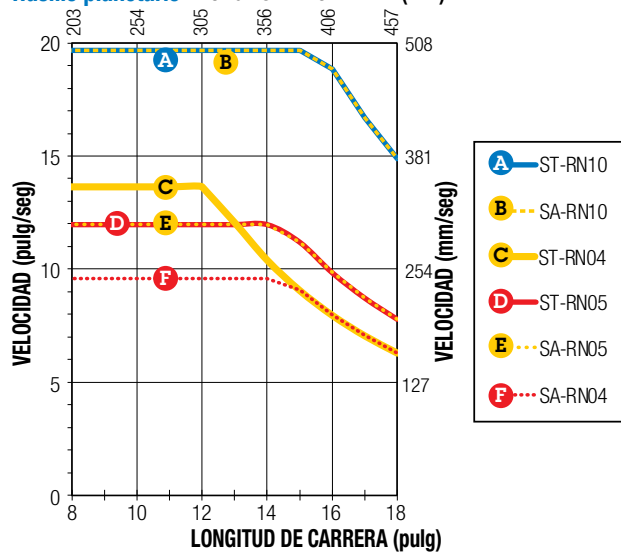
Husillo planetario LONGITUD DE CARRERA (mm)
